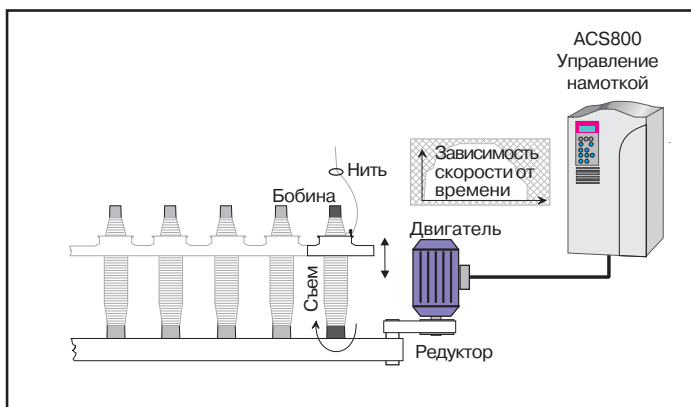
Принцип управления намоткой.
