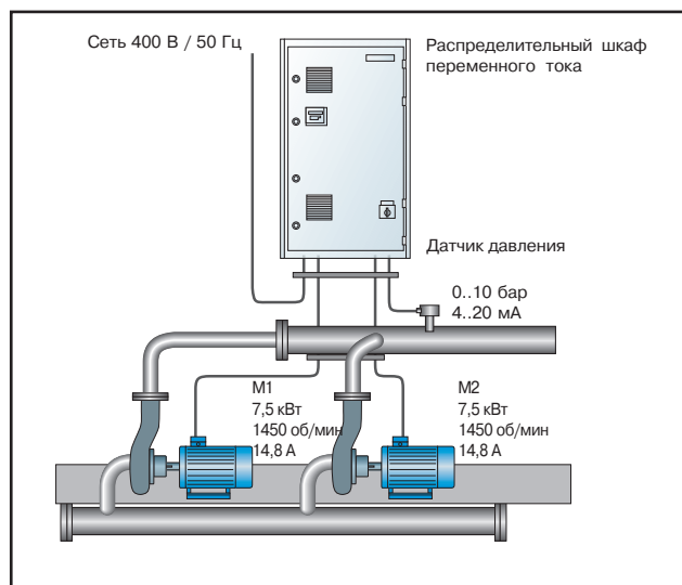
Насосная станция с двумя насосами. Привод ACS800 установлен внутри распределительного шкафа.
