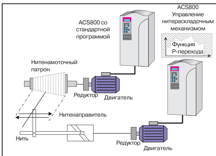
Принцип управления нитераскладочным механизмом.
