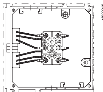
Terminal box size 112-132.
