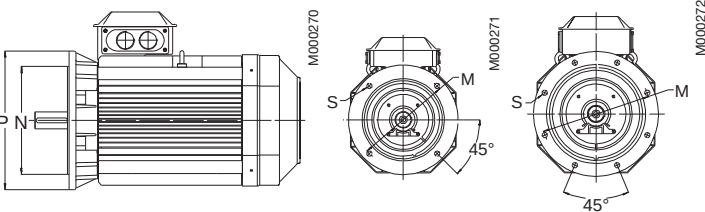
Foot-mounted motor IM 3001 / B5
