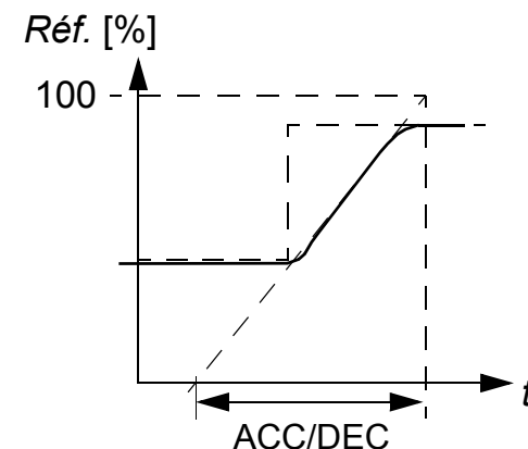
Temps ACC/DEC
