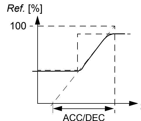
Tempo ACC/DEC
